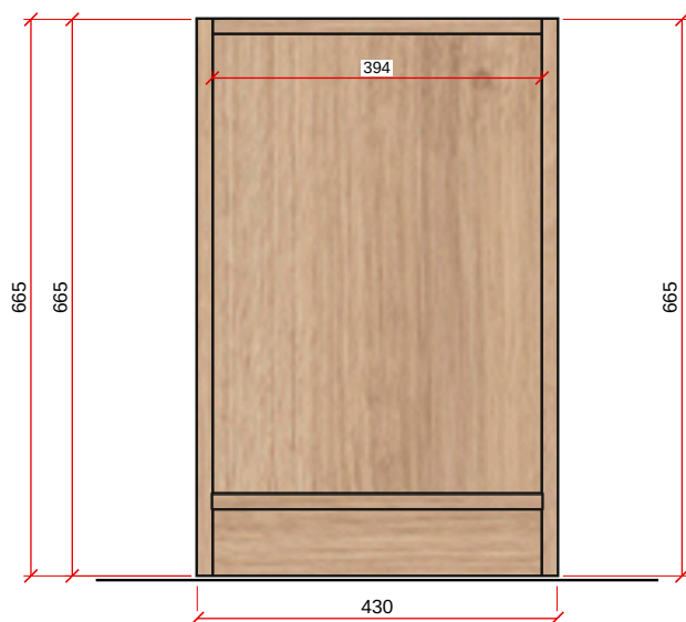
VISTA C - ESC. 1:10
