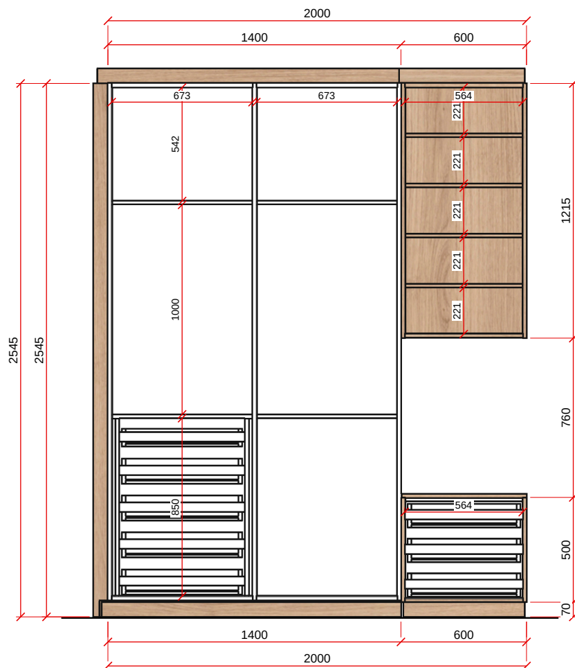
VISTA A - ESC. 1:25
