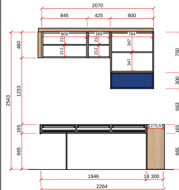
VISTA B - ESC. 1:40
